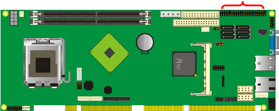
CN_USB1/2/3/4
