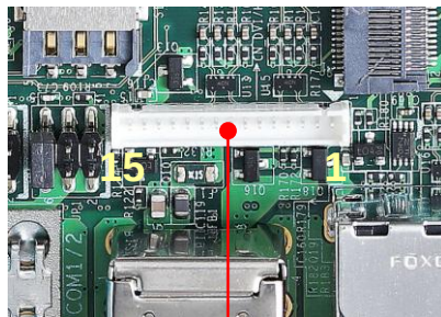
CN_DVI/HDMI
