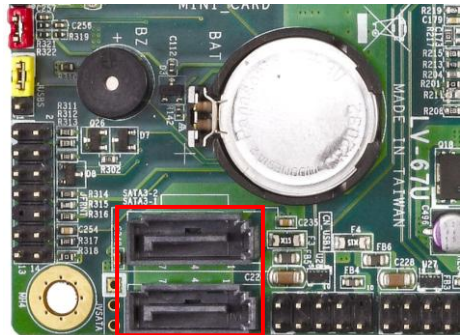
SATA3-2
